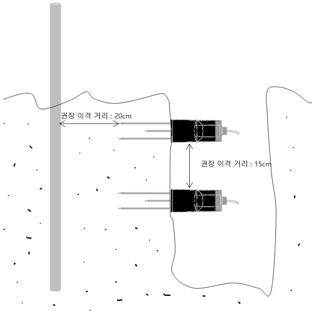
[설치 예제 4.]
