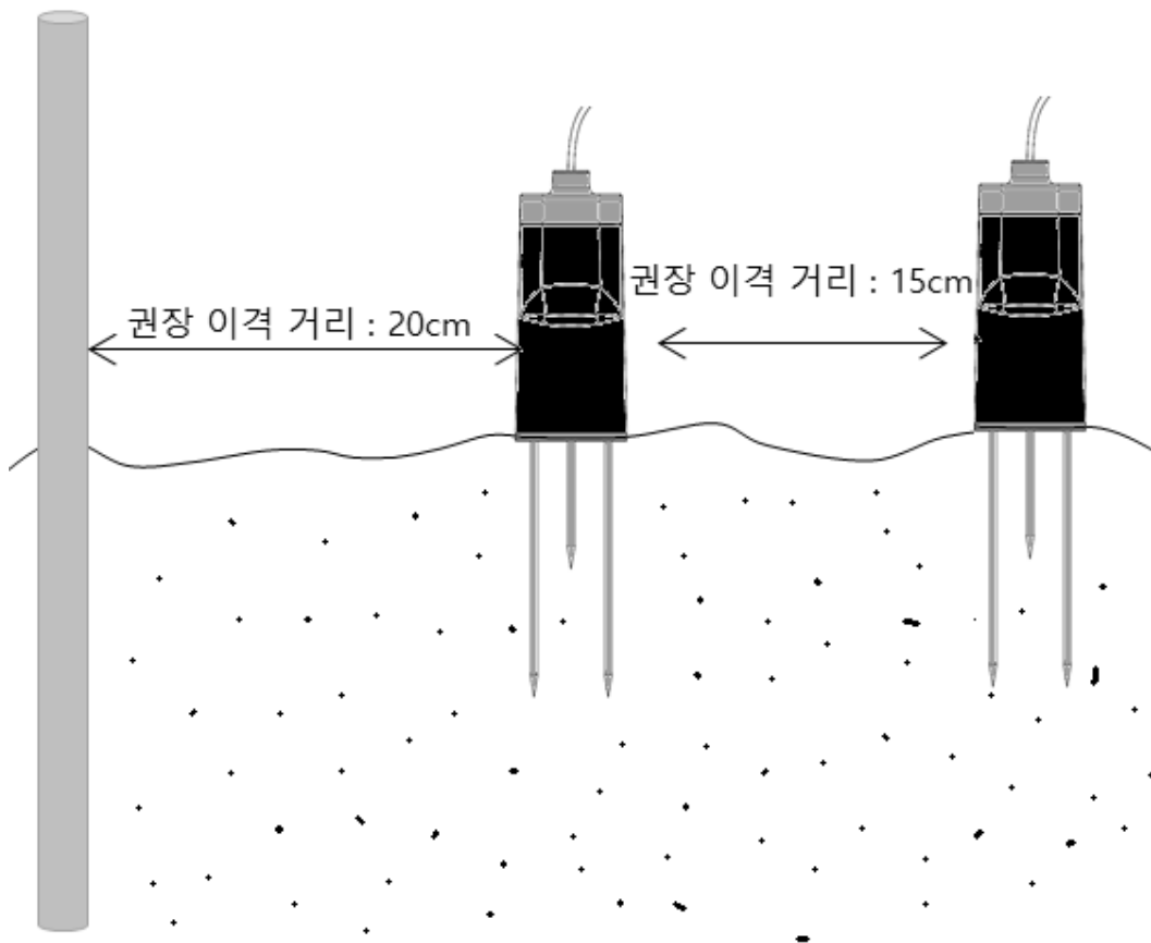
[설치 예제 3.]
